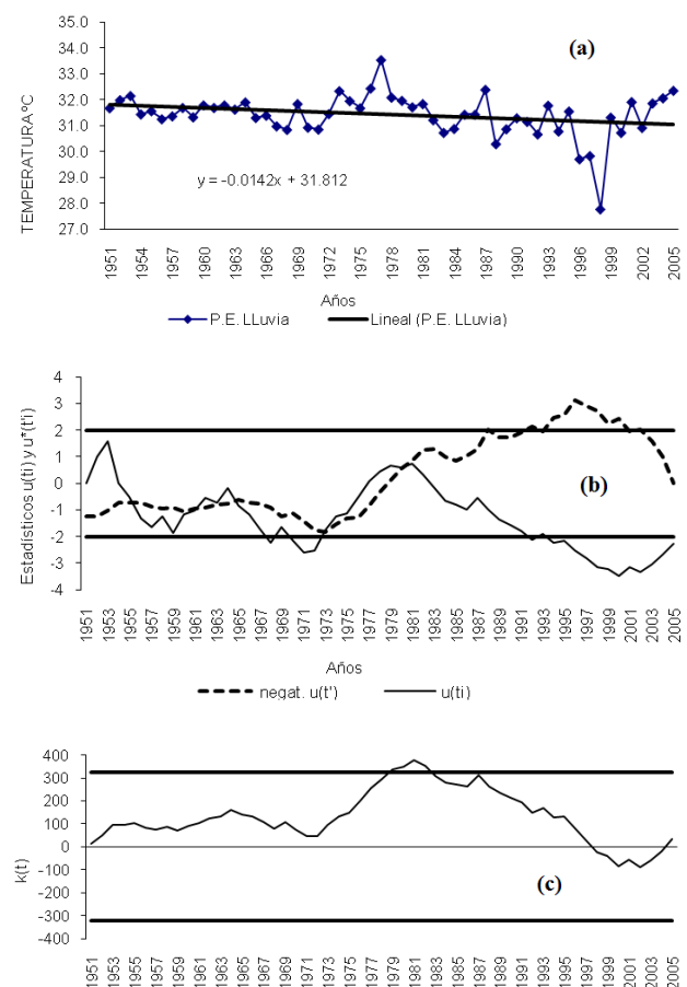
Figura 7. Temperatura Máxima de la Época Lluviosa (a) Regresión lineal, (b) Estadígrafos u^*(t) , de la Prueba de Mann – Kendall, (c) Estadígrafo k(t) de la prueba de Pettitt. Las líneas horizontales representan el intervalo de confianza del 95%.
