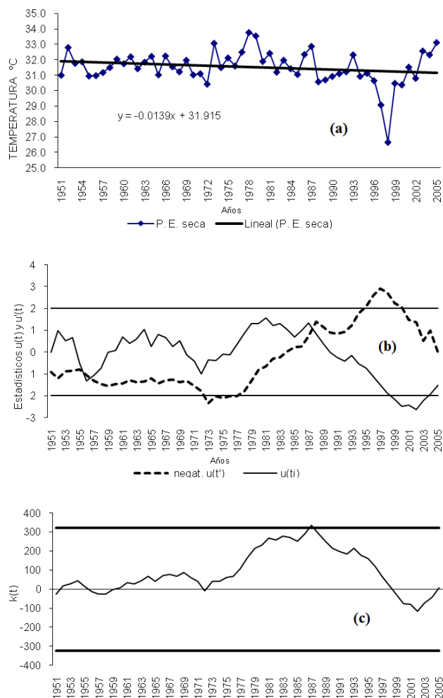
Figura 6. Temperatura Máxima de la Época Seca (a) Regresión lineal, (b) Estadígrafos u^*(t) , de la Prueba de Mann – Kendall, (c) Estadígrafo k(t) de la prueba de Pettitt. Las líneas horizontales representan el intervalo de confianza del 95 %.
