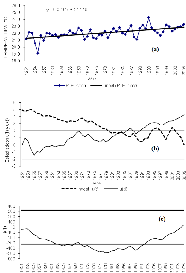
Figura 9. Temperatura Mínima de la Época Seca (a) Regresión lineal, (b) Estadígrafos u^*(t_i) , de la Prueba de Mann – Kendall, (c) Estadígrafo k(t) de la prueba de Pettitt. Las líneas horizontales representan el intervalo de confianza del 95%.
