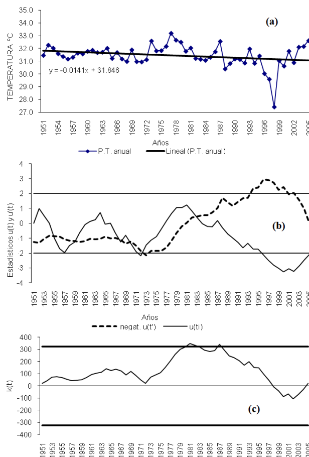
Figura 5. Temperatura Máxima Total Anual (a) Regresión lineal, (b) Estadígrafos u^*(t) , de la Prueba de Mann – Kendall, (c) Estadígrafo k(t) de la prueba de Pettitt. Las líneas horizontales representan el intervalo de confianza del 95%.
