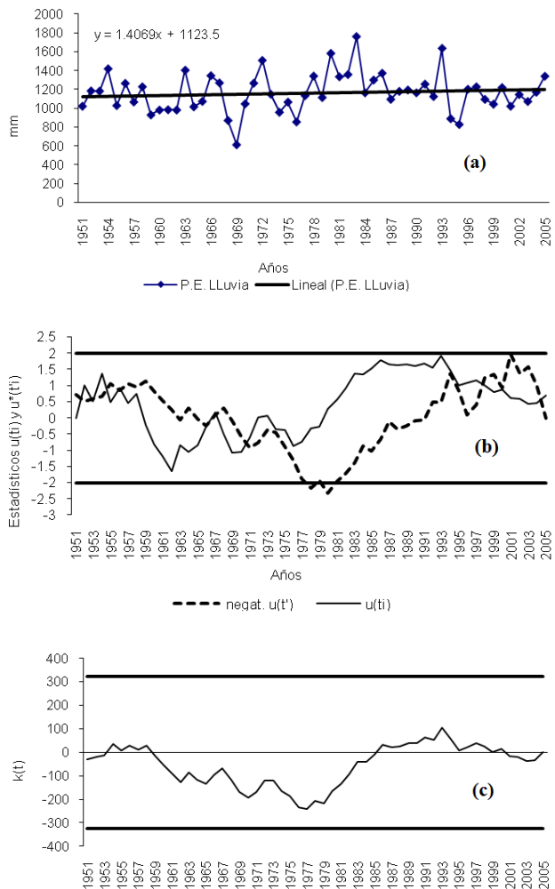
Figura 4. Precipitación de la Época de Lluvia. (a) Regresión lineal, (b) Estadígrafos u^*(t_i) , de la Prueba de Mann – Kendall, (c) Estadígrafo k(t) de la prueba de Pettitt. Las líneas horizontales representan el intervalo de confianza del 95%
