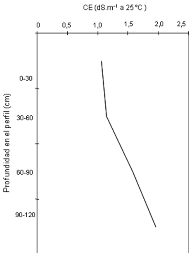
Figura 3. Comportamiento de la conductividad eléctrica (CE) en relación a la profundidad de los suelos en el sector Caño San Miguel, municipio Mara, estado Zulia, Venezuela.
