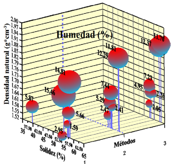
Figura 6. Densidad aparente natural versus la relación de solidez, los métodos de medición (Densímetro (1), Uhland libre (2) y Uhland forzado (3)) y la humedad del suelo en tres tipos de suelos del estado Monagas.
