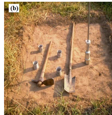
Figura 2. Equipos utilizados en las evaluaciones: (a) densímetro nuclear HS-5001C y b) Toma de muestras tipo Uhland H-4203.3
