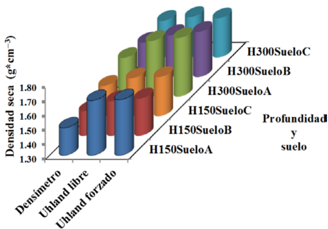
Figura 5. Densidad aparente seca obtenidas por los tres métodos en las dos profundidades de los tres suelos estudiados del estado Monagas.
