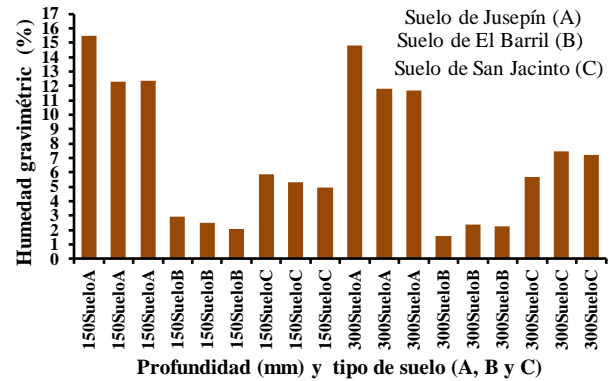
Figura 3. Contenido de humedad gravimétrica in situ de los tres tipos de suelos del estado Monagas al momento de la evaluación
